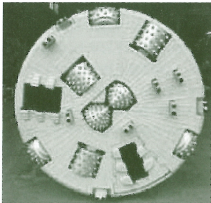
写真一三 マルチカッタヘッド
