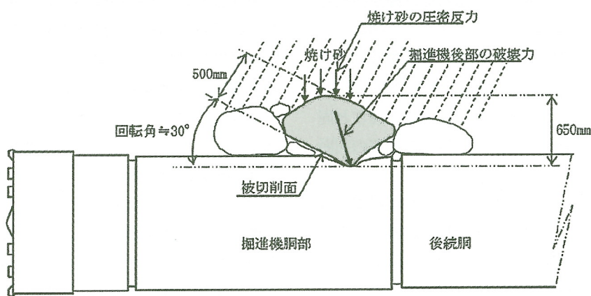
図-2 玉石のカム作用の模式図
