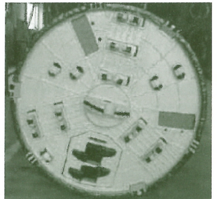
写真一五 切削カッタヘッド
