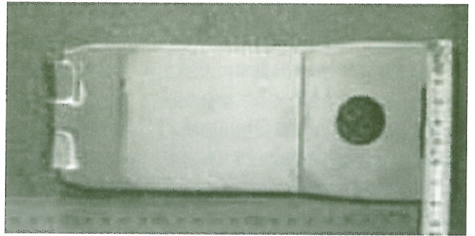
写真-2 ローラビットと切削ビット
