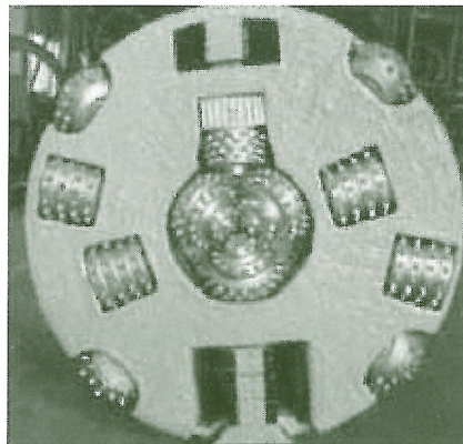
写真一四 ローラカッタヘッド
